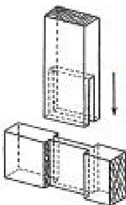
Enfourchement en T
