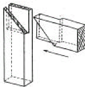
Enfourchement d'onglet
